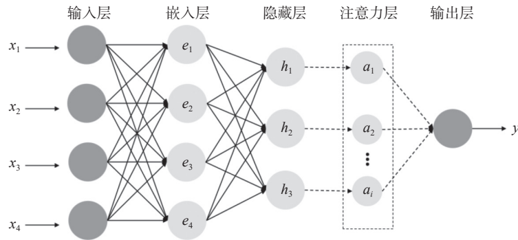
图2 神经网络结构图
